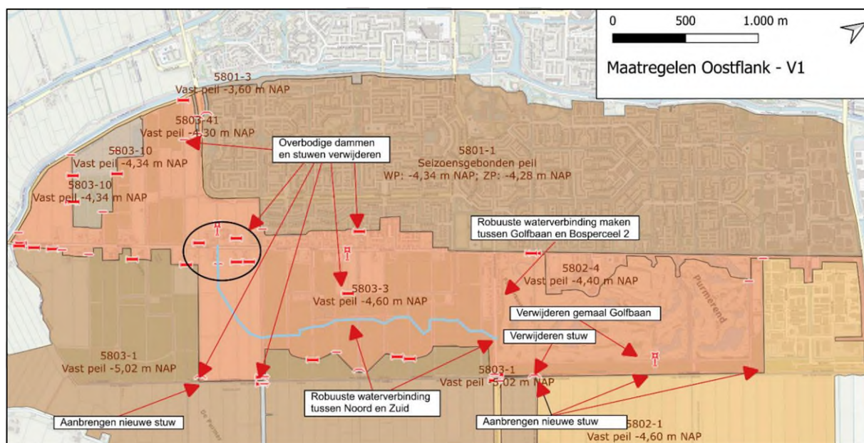
Figuur 10-2 Te nemen maatregelen m.b.t. peilgebied variant 1. (bron: Watervarianten Oostflank. Sweco, 2025)
