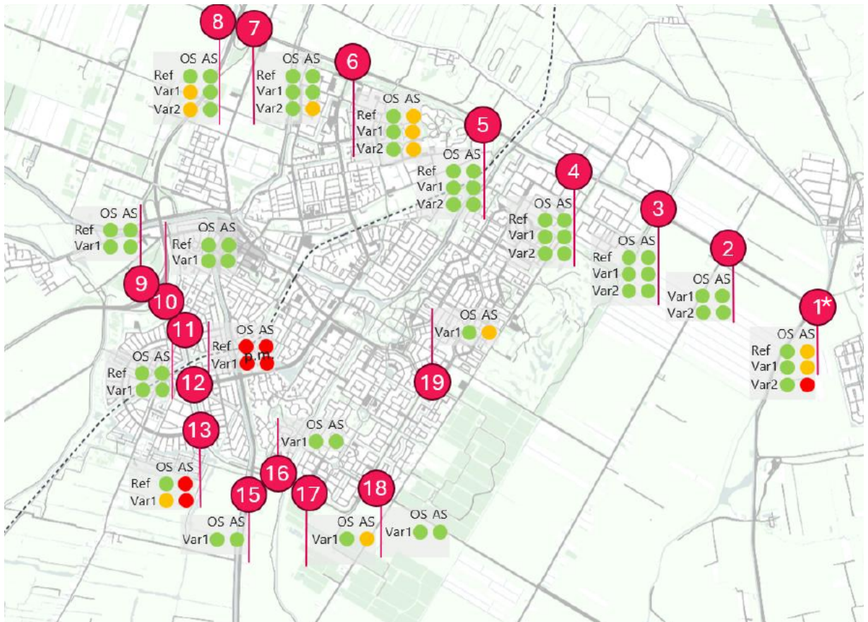
Figuur 15-6 Kruispuntbelastingen verkeersvarianten 1 en 2 inclusief voorgestelde infrastructurele maatregelen (bron: Goudappel, 2025) Verkeersvariant 2 is gelijk aan het voorkeursalternatief
