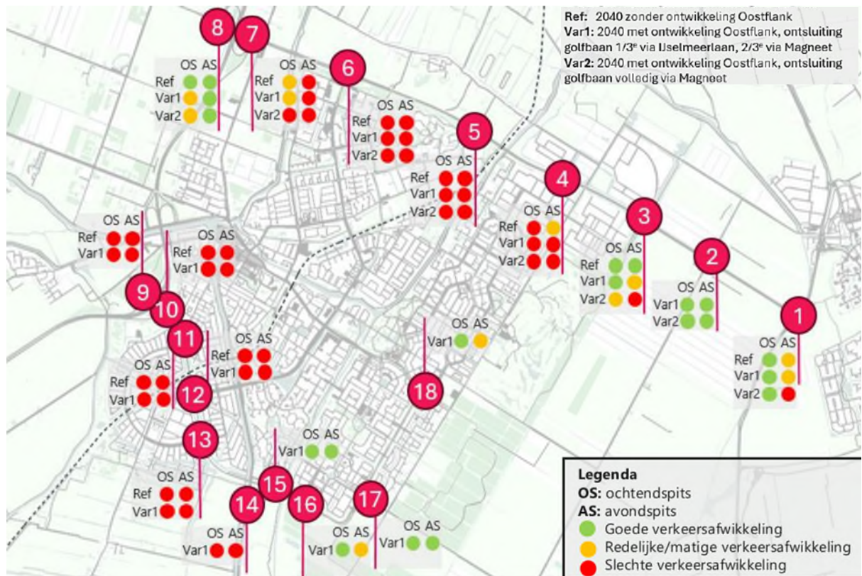
Figuur 8-14 Kruispuntbelastingen verkeersvarianten 1 en 2 t.o.v. referentiesituatie 2040
