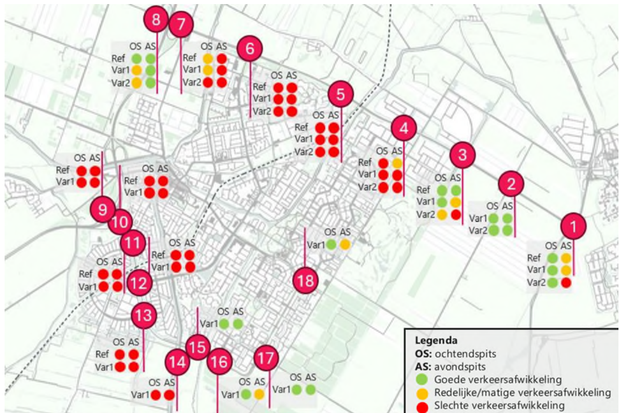
Figuur 15-5 Kruispuntbelastingen verkeersvarianten 1 en 2 t.o.v. referentiesituatie 2040 (bron: Goudappel, 2025) Verkeersvariant 2 is gelijk aan het voorkeursalternatief
