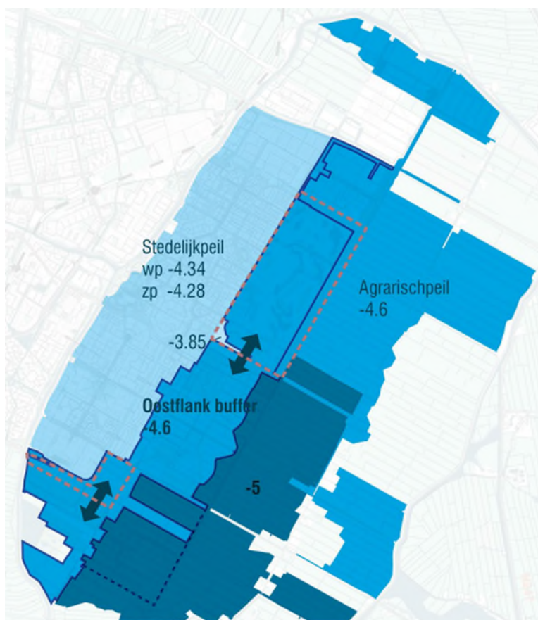
Figuur 10-3 Schematische weergave beoogde peilsysteem variant 1 (bron: West8, 2025)
